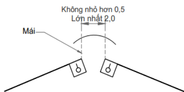
(f) Dầm nóc có thông gió
