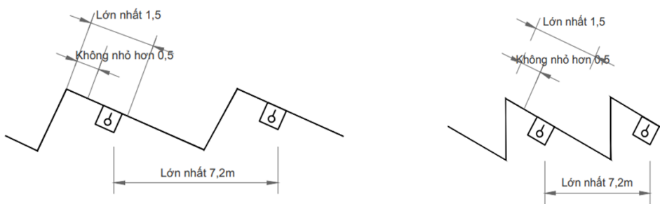
(a) Bề mặt dốc khác nhau
