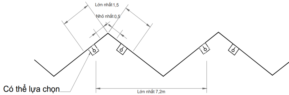
(c) Bề mặt dốc như nhau
