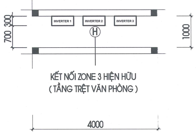
MẶT BẰNG HỆ THỐNG BÁO CHÁY
